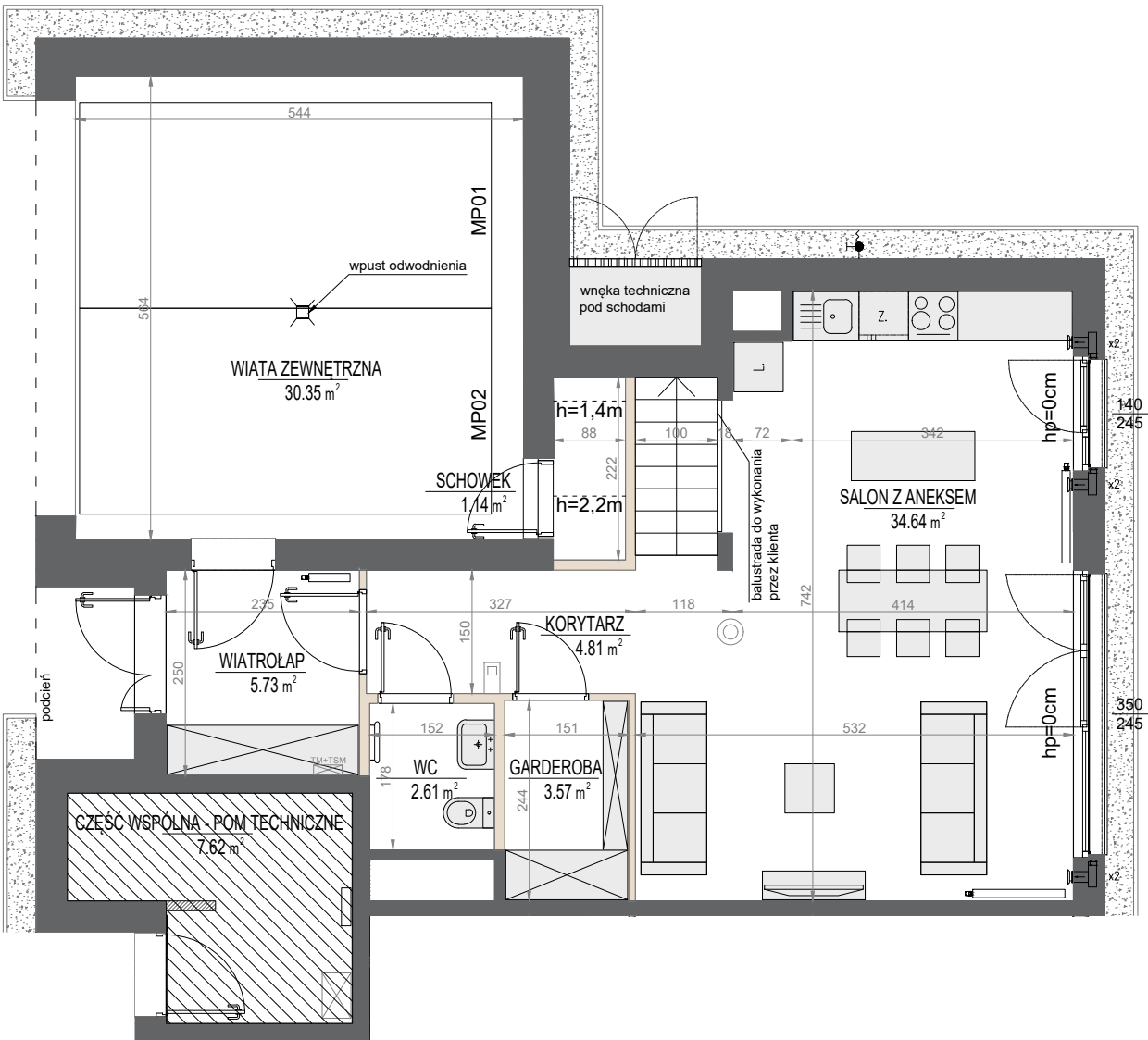
RZUT PARTERU
